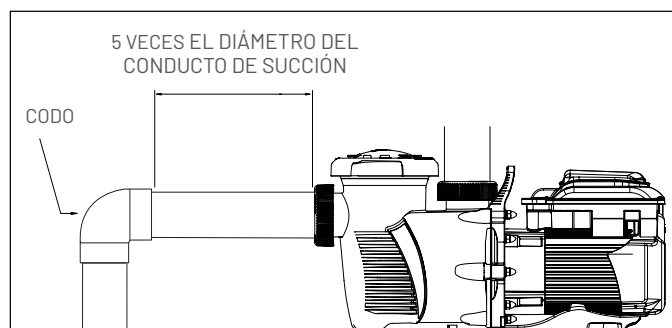
Figura 2: Conductos recomendados
